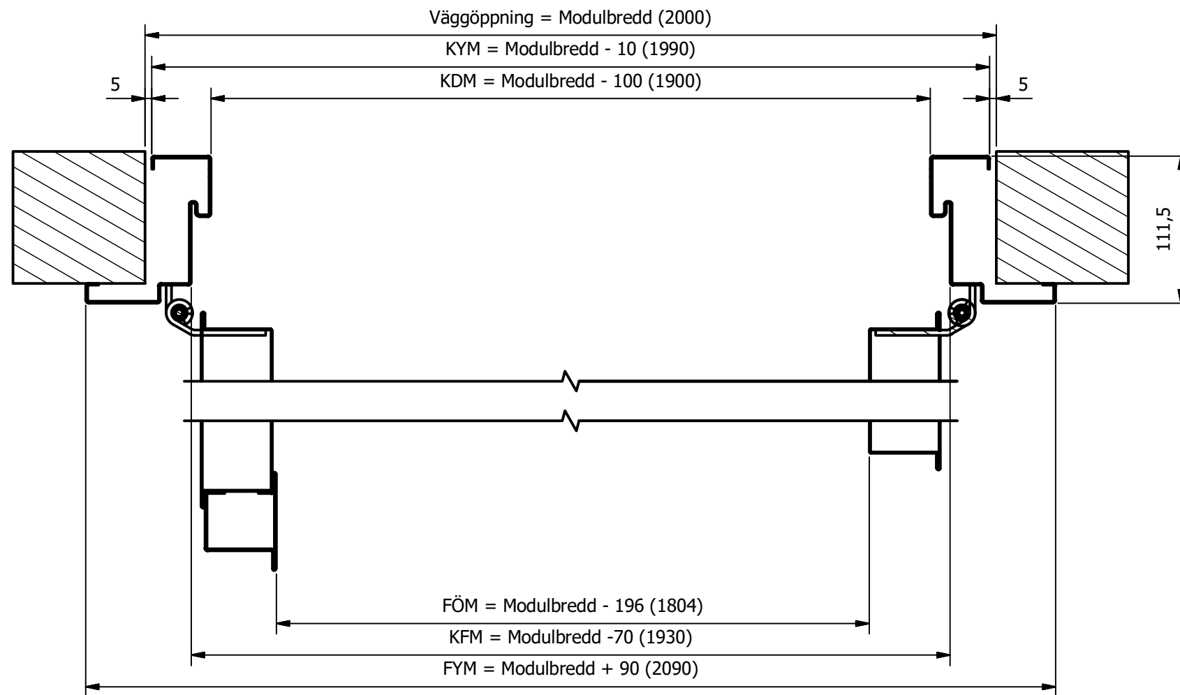
A (1 : 2)
